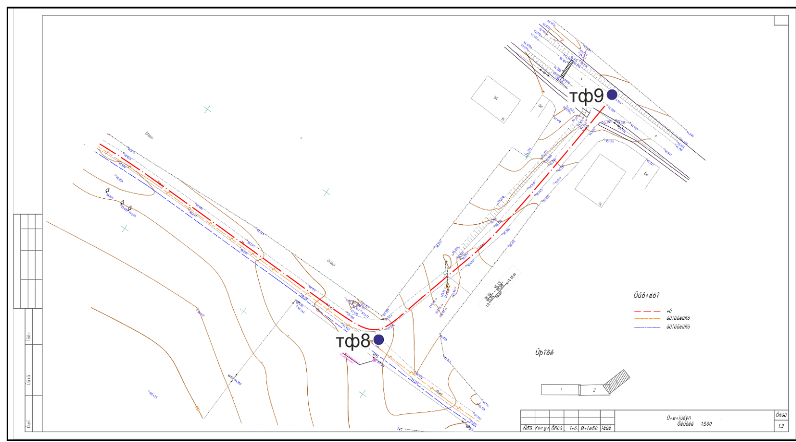
Рис. 7. Объект «Строительство автомобильной дороги по улицам Новая и Северная, в с. Байдеряково Яльчикского района Чувашской Республики». Схема отводимого земельного участка с рекогносцировочным шурфом и точками фотофиксации на топографической основе, предоставленной заказчиком исследований. Лист 3.
