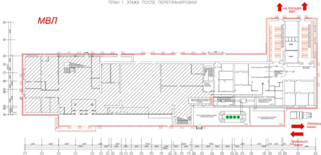
ПЛАН 1 ЭТАЖА ПОСЛЕ ПЕРЕПЛАНИРОВКИ
