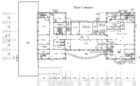
План 1 этажа
