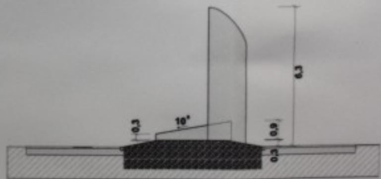
надрез 1 : 100
