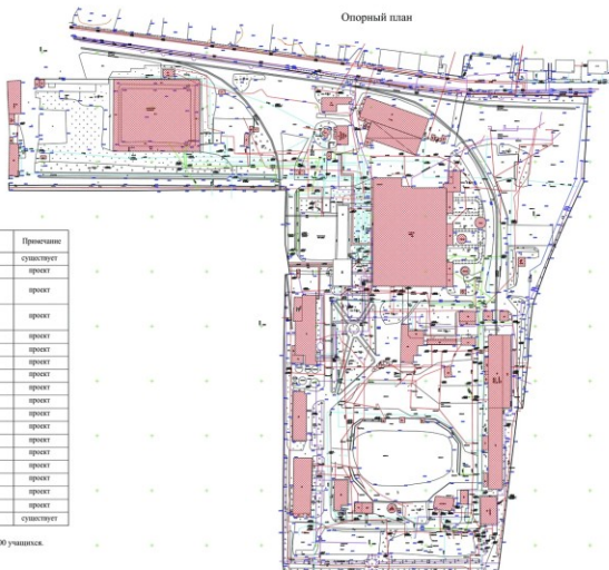
Опорный план
