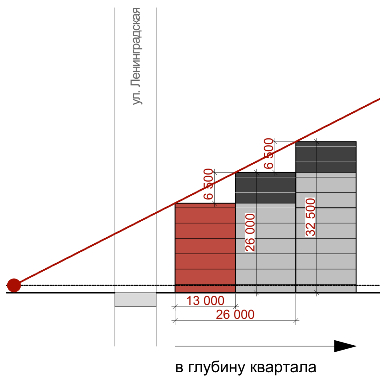
Контрольное сечение при высоте ОКН по красной линии 5 этажей
