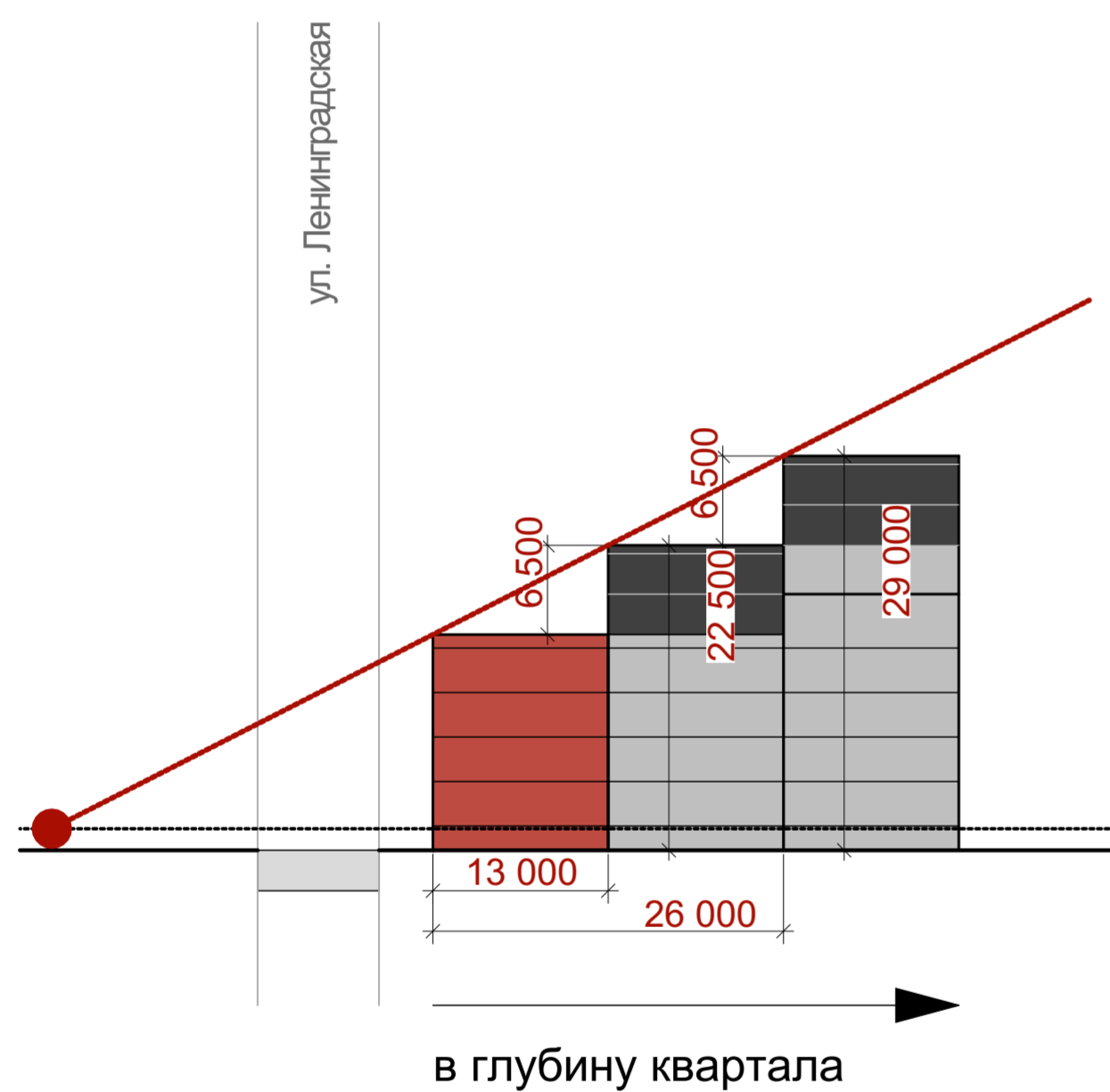
Контрольное сечение при высоте ОКН по красной линии 4 этажа
