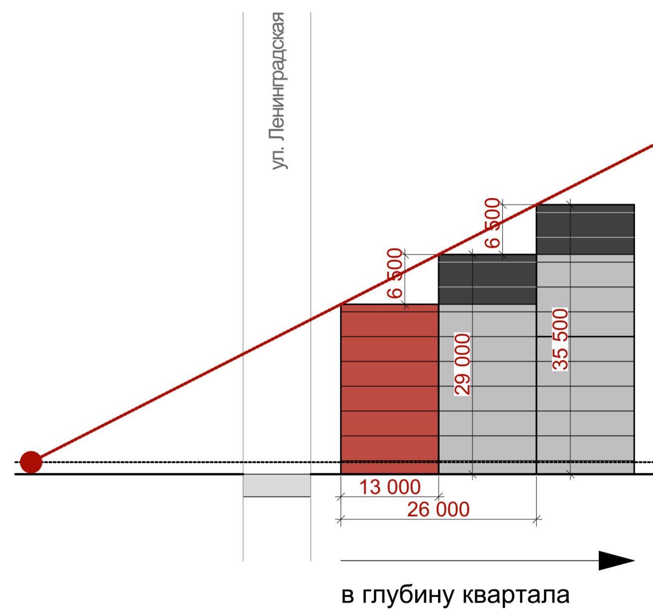
Контрольное сечение при высоте ОКН по красной линии 6 этажей
