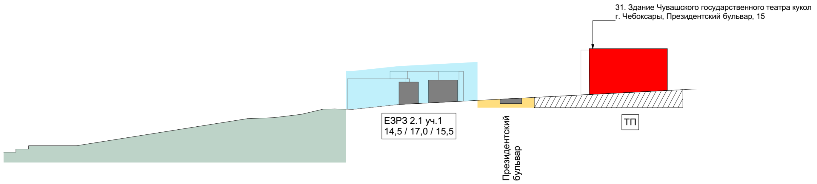
Контрольное сечение 2-2
