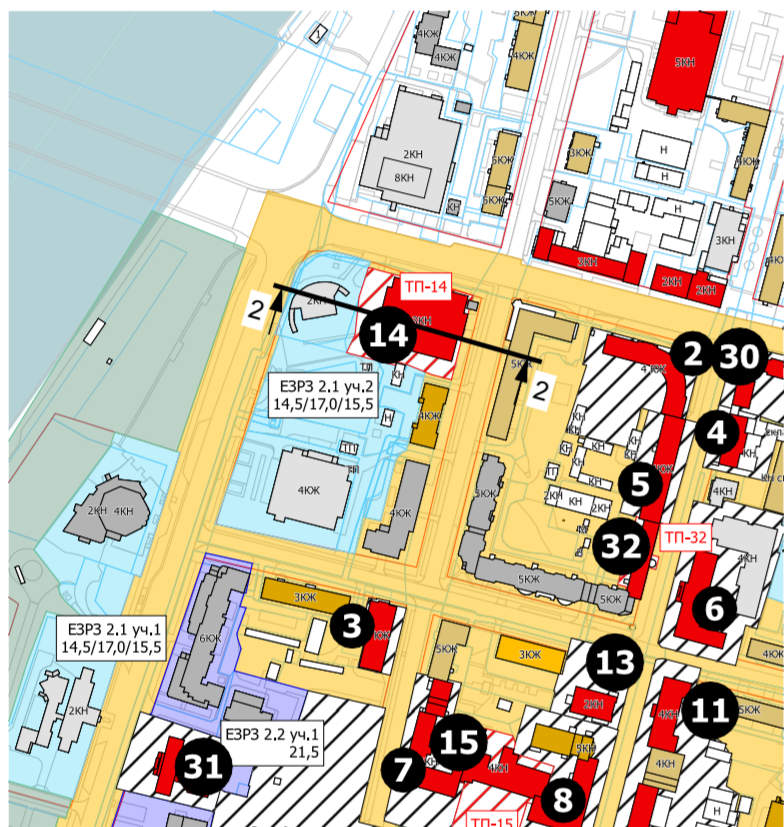
Контрольное сечение 2-2
