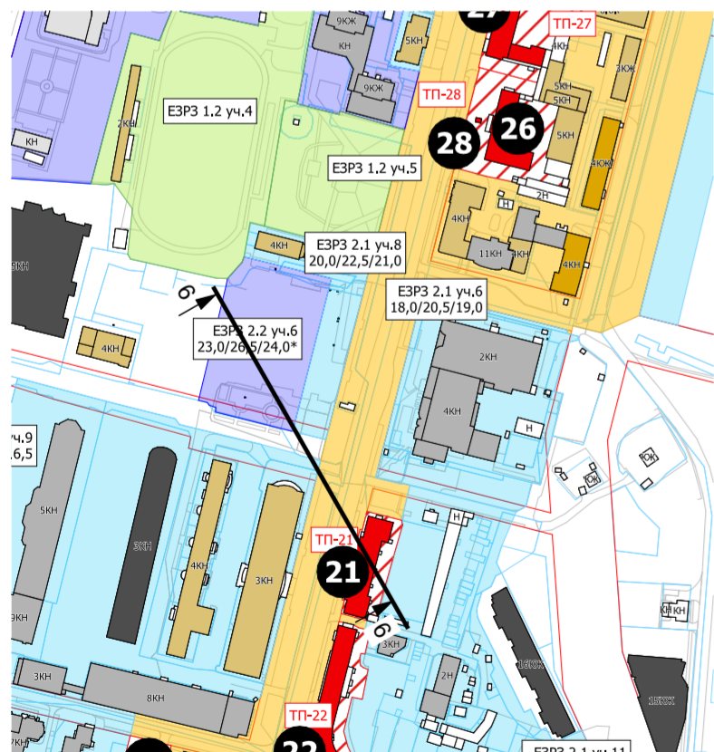
Контрольное сечение 6-6
