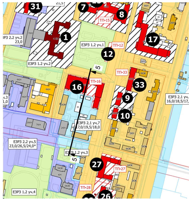
Контрольное сечение 5-5
