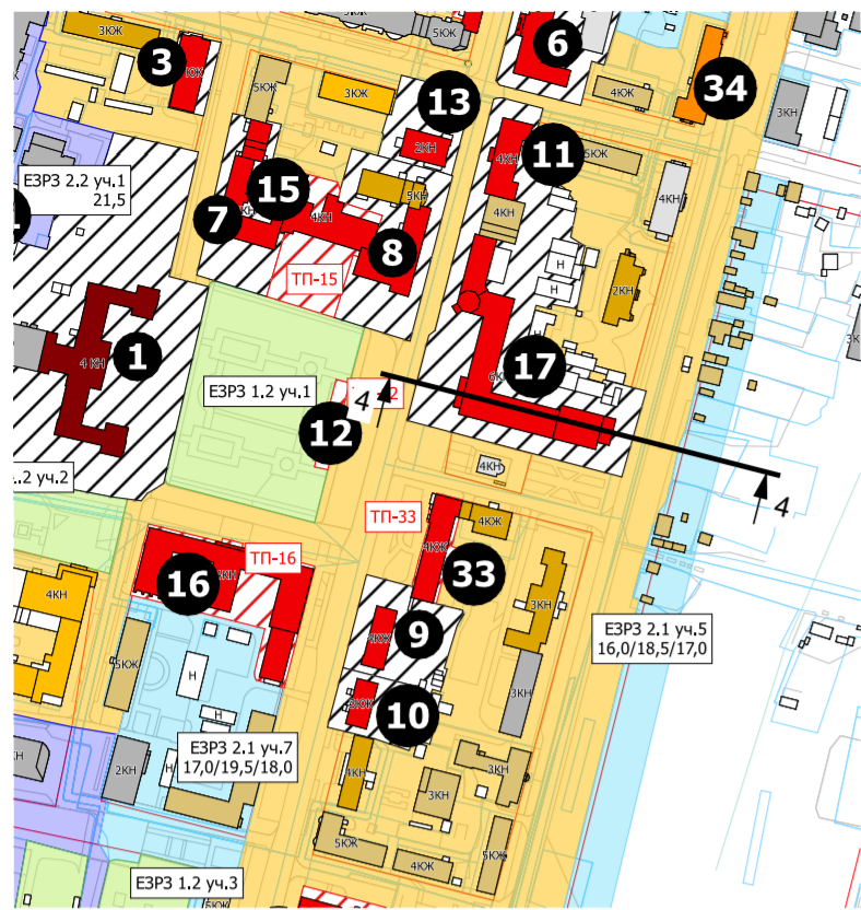
Контрольное сечение 4-4
