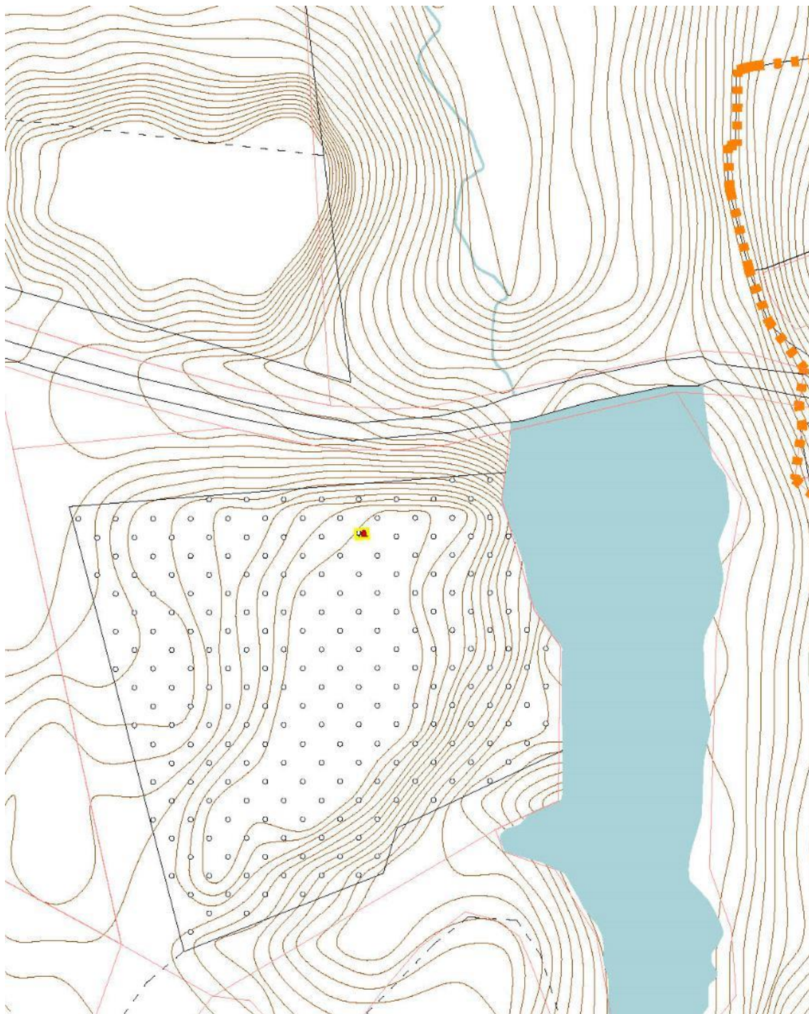
Схема актуализированной геоподосновы территории исследования
