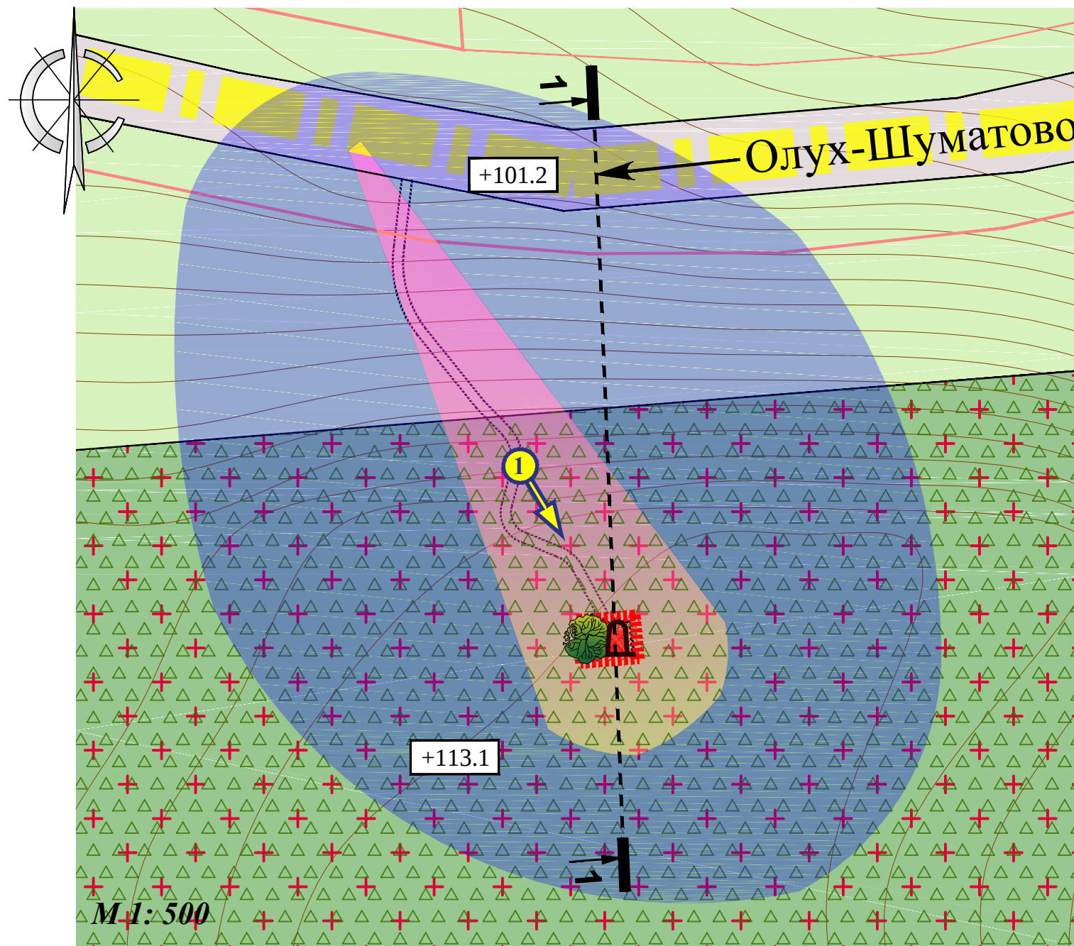
Сечение 1-1
