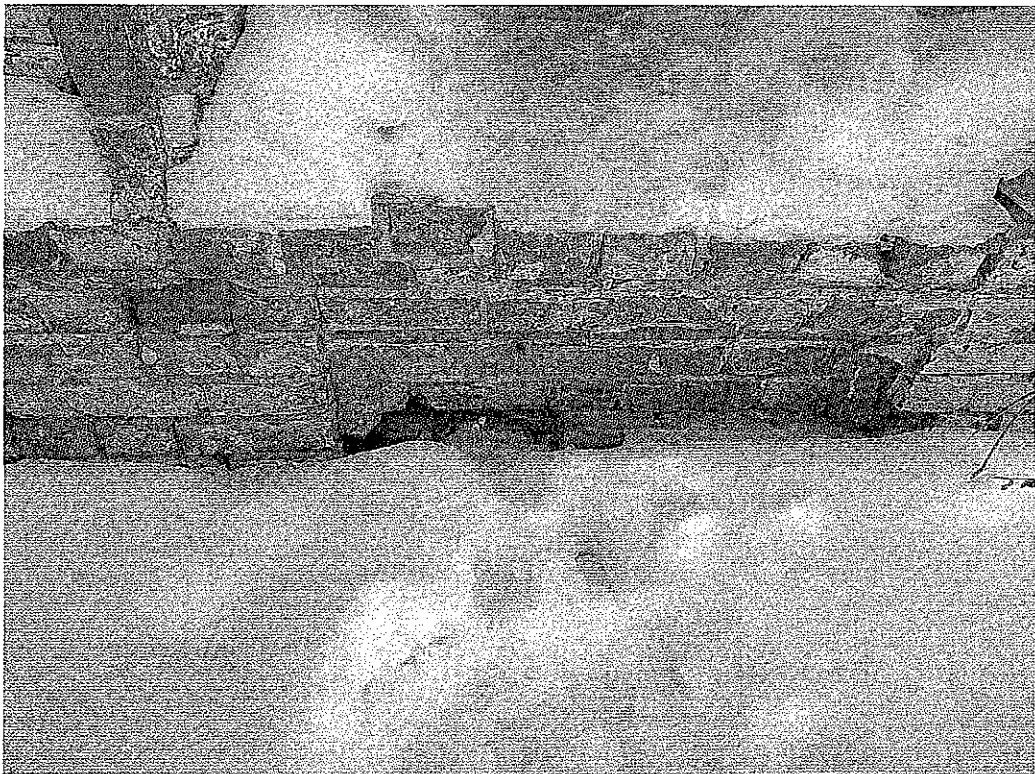
Фото 6. Выпадение кирпича.
