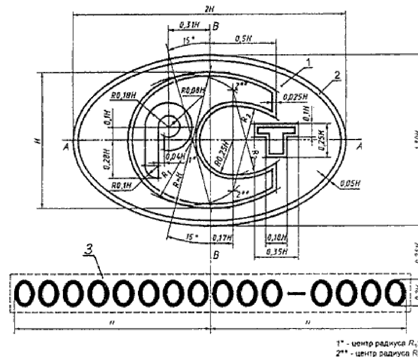
РАЗМЕРЫ знака национальной системы стандартизации
